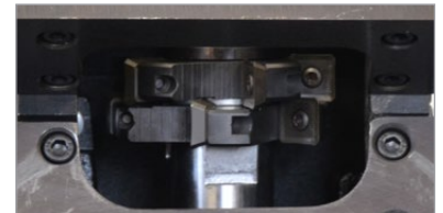
2 roterende freeskoppen met elk vijf 4-zijdige wisselplaten
