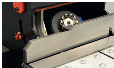
Eenvoudig toegang tot de freoskop en beitelplaten
